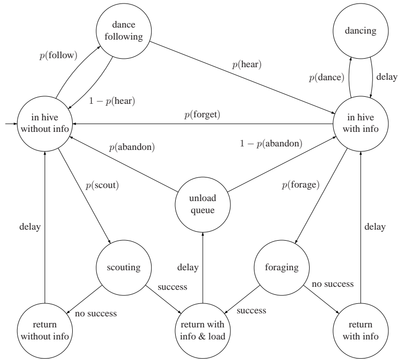
Abbildung 1: Zustandsmodell einer Honigbiene aus (SC04)
