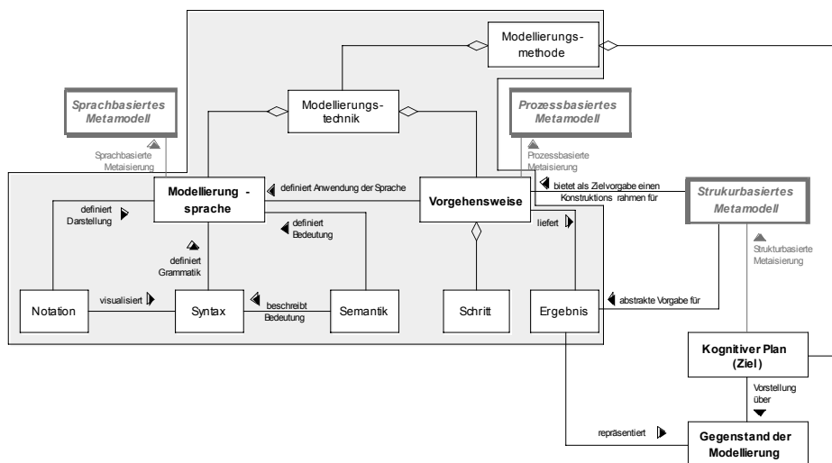
Abbildung 1: Metamodell einer Modellierungsmethode
