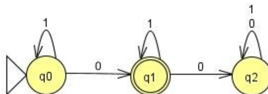
Abbildung 3: DEA für L1 .
